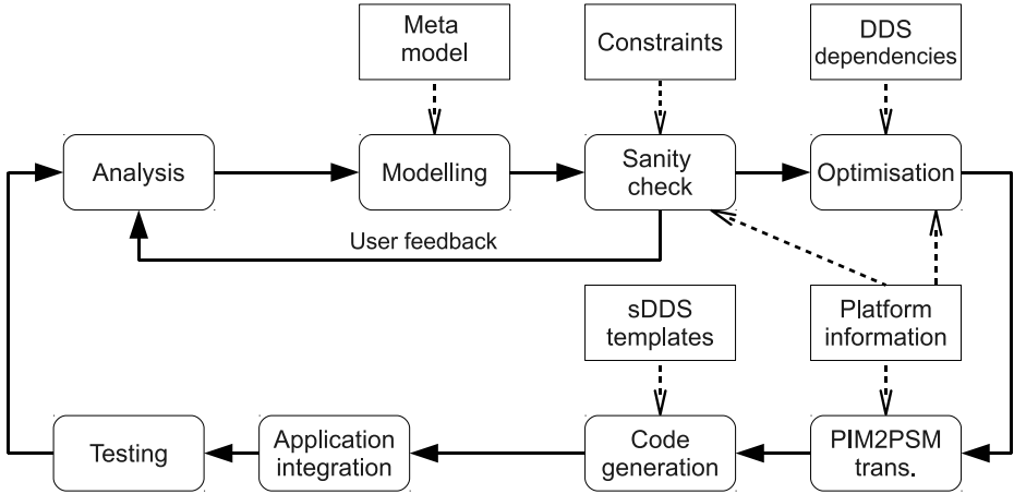
Fig. 3. MDSM workflow
